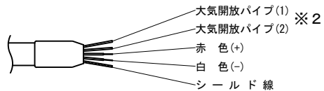
A部ケーブル接続図 S=NON
