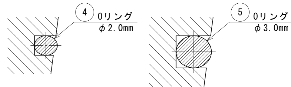
A部詳細図 S=5/1
