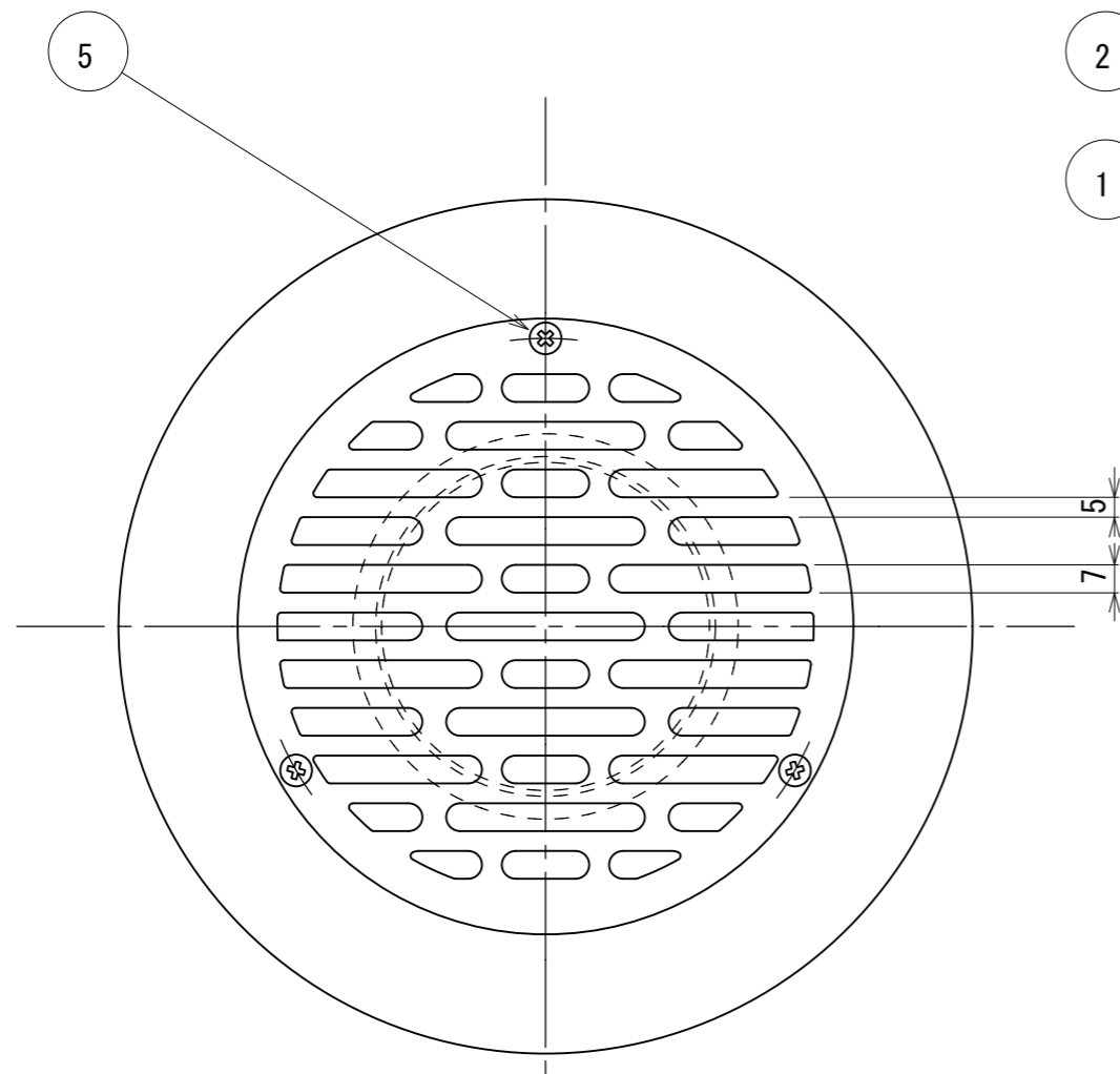
平面図
