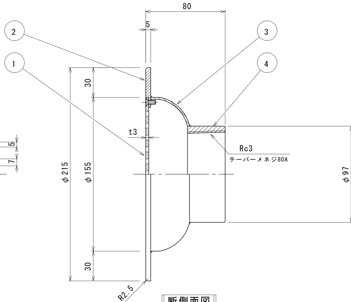
断側面図
