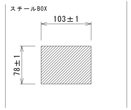
制御盤への取付時の開口寸法 S=1/4
