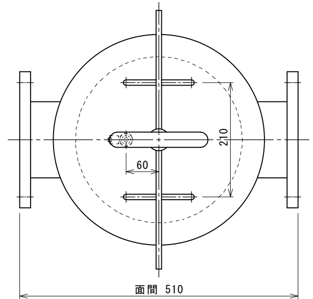
A 矢視図
