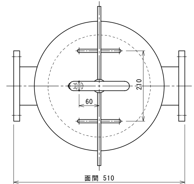
A 矢視図
