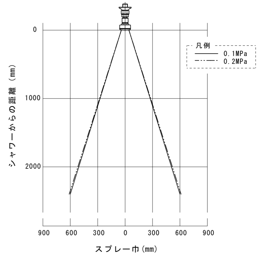
天井取付時のスプレーパターン
