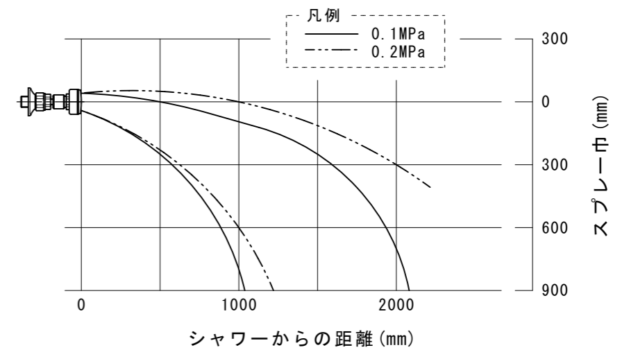
壁面取付時のスプレーパターン
