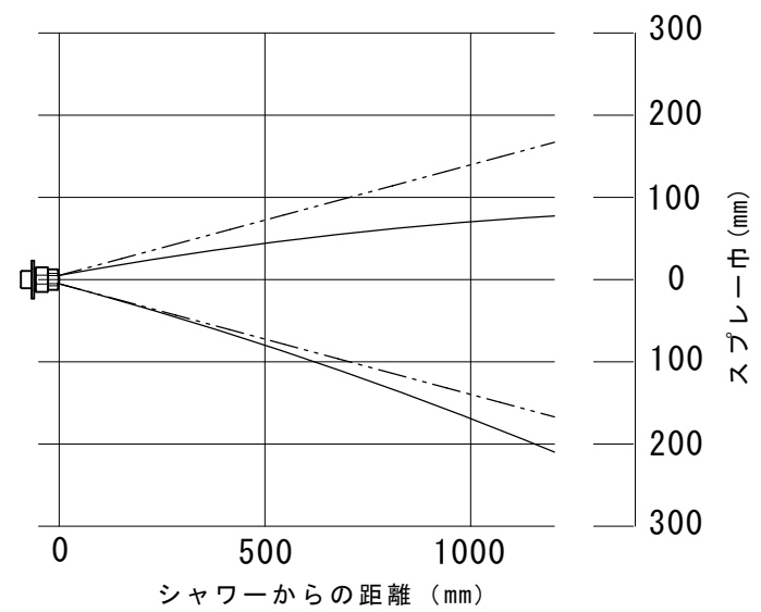
△ 壁取付時のスプレーパターン
