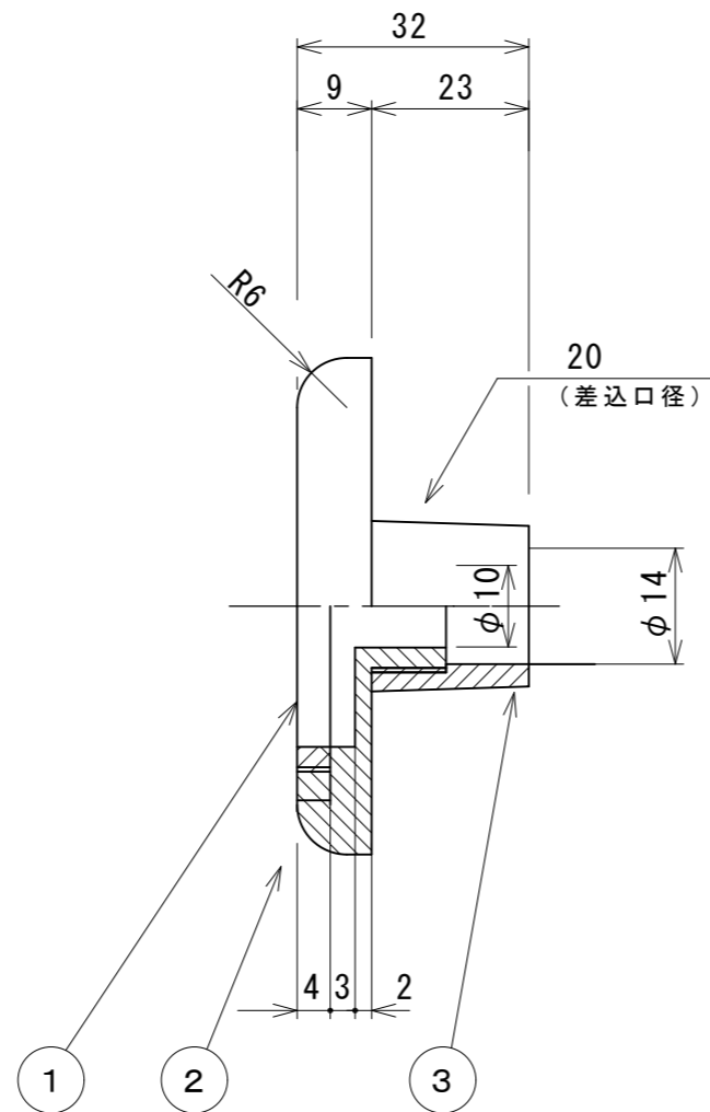
断側面図
