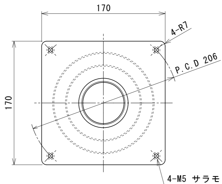
B 矢視図
