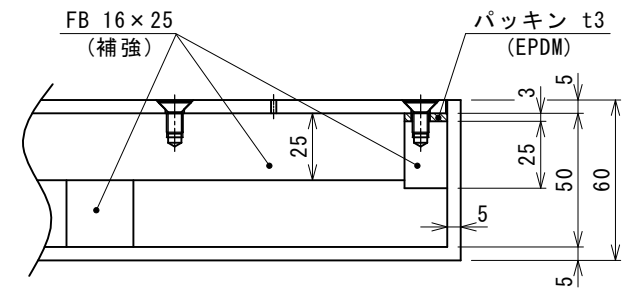
端部詳細図 S=1/2
