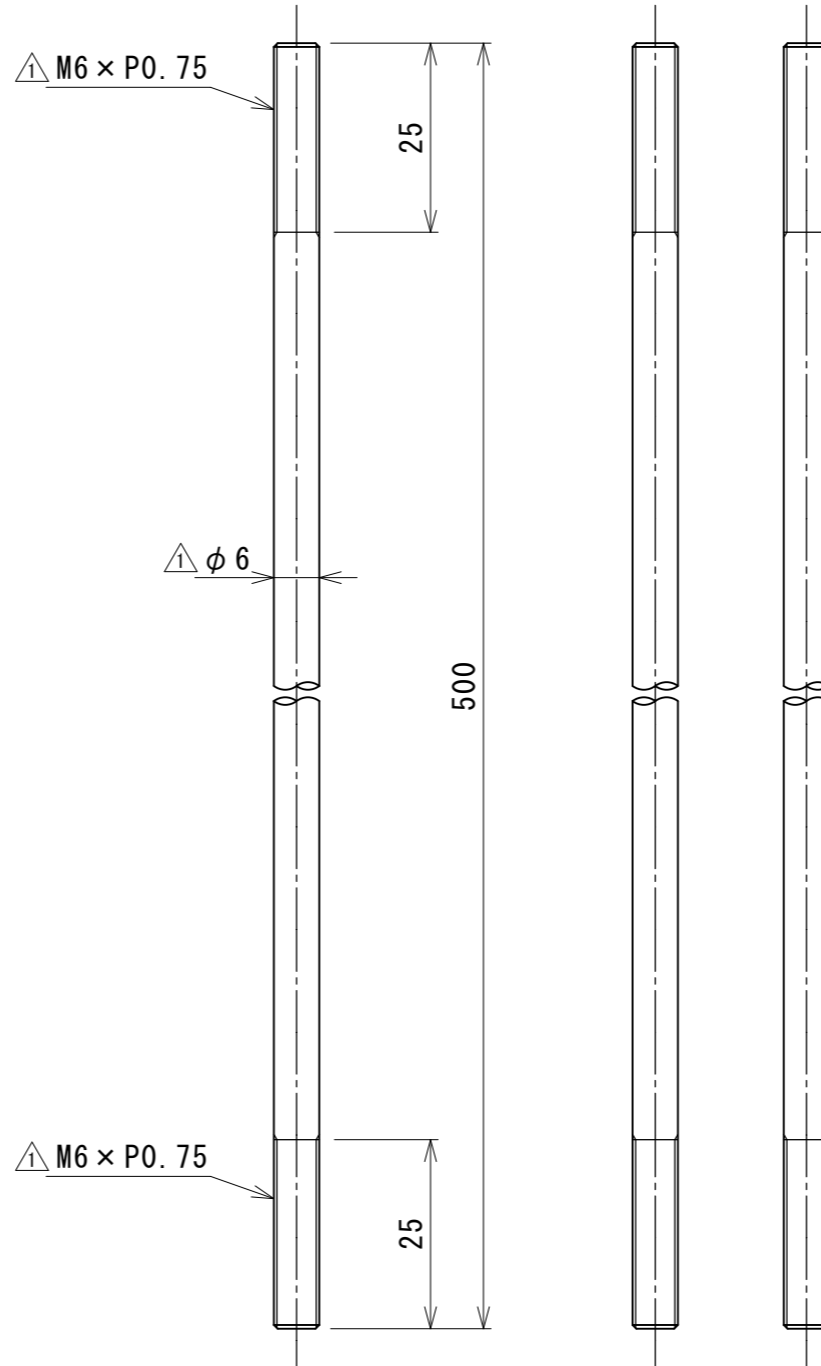
8 電極棒 S=1/1
