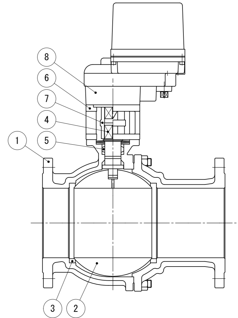
部品名称図 S=NON
