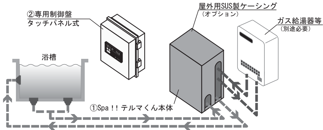
※上記フロー図は標準品ZX-SDHシリーズのイメージとなります。
