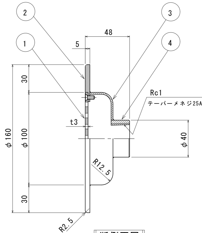
断側面図
