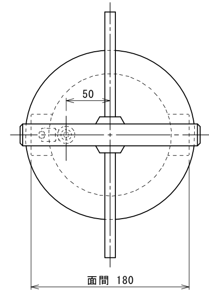
A 矢視図
