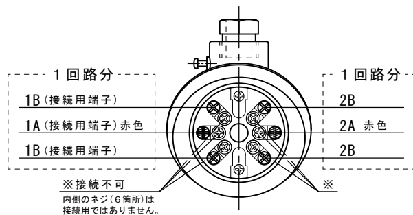
配線図 (2回路型)
