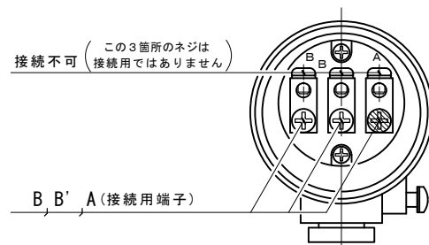
配線図
