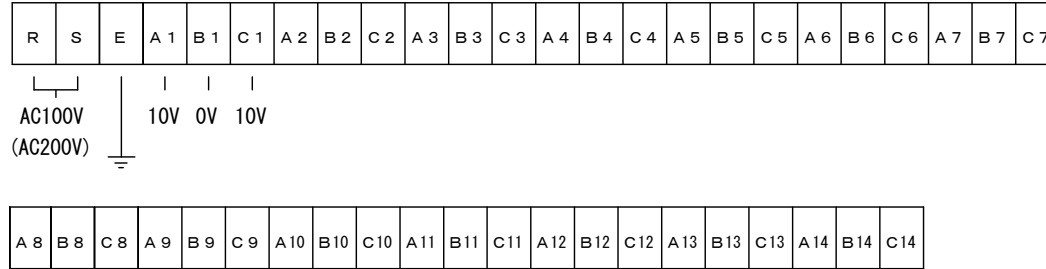
端子図 (例TB-14)
