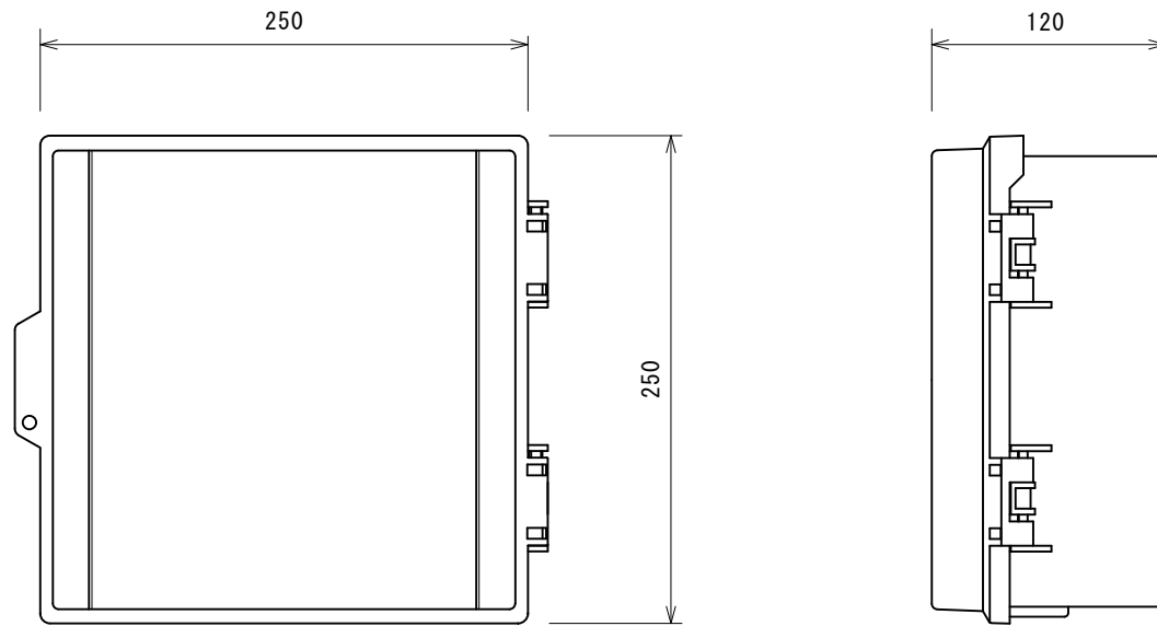
制御BOX プラスチック P12-2525
