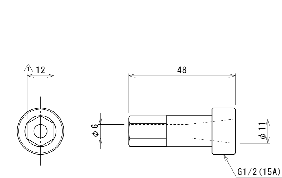
3 内部ノズル
