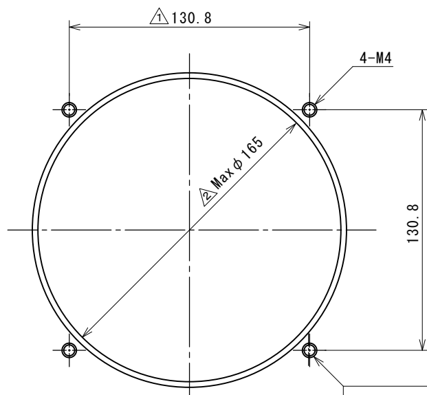
取付寸法
