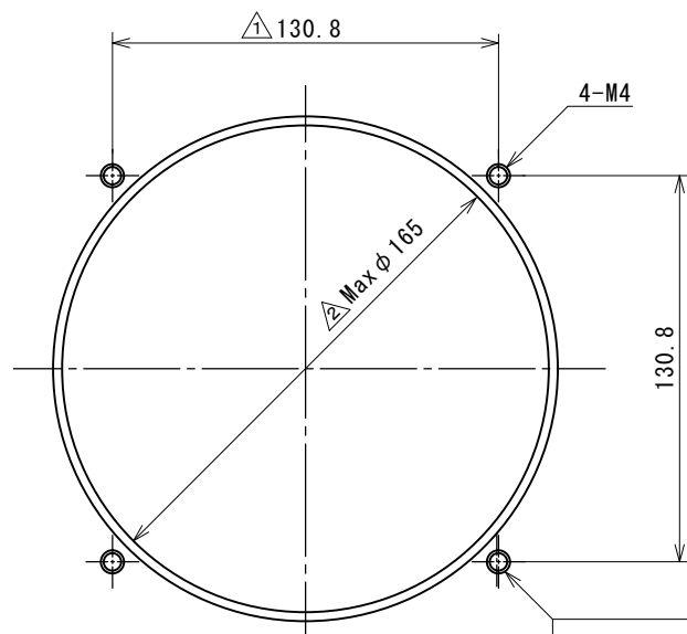
取付寸法
