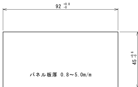
パネル切穴
