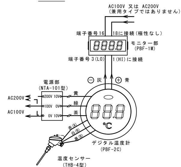
結線図
