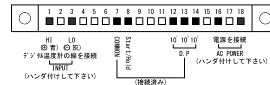
端子台図
