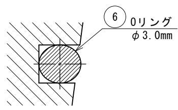
C 部詳細図 S=5/1
