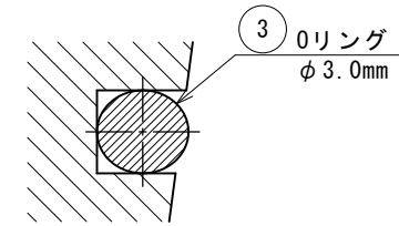
A部詳細図 S=5/1
