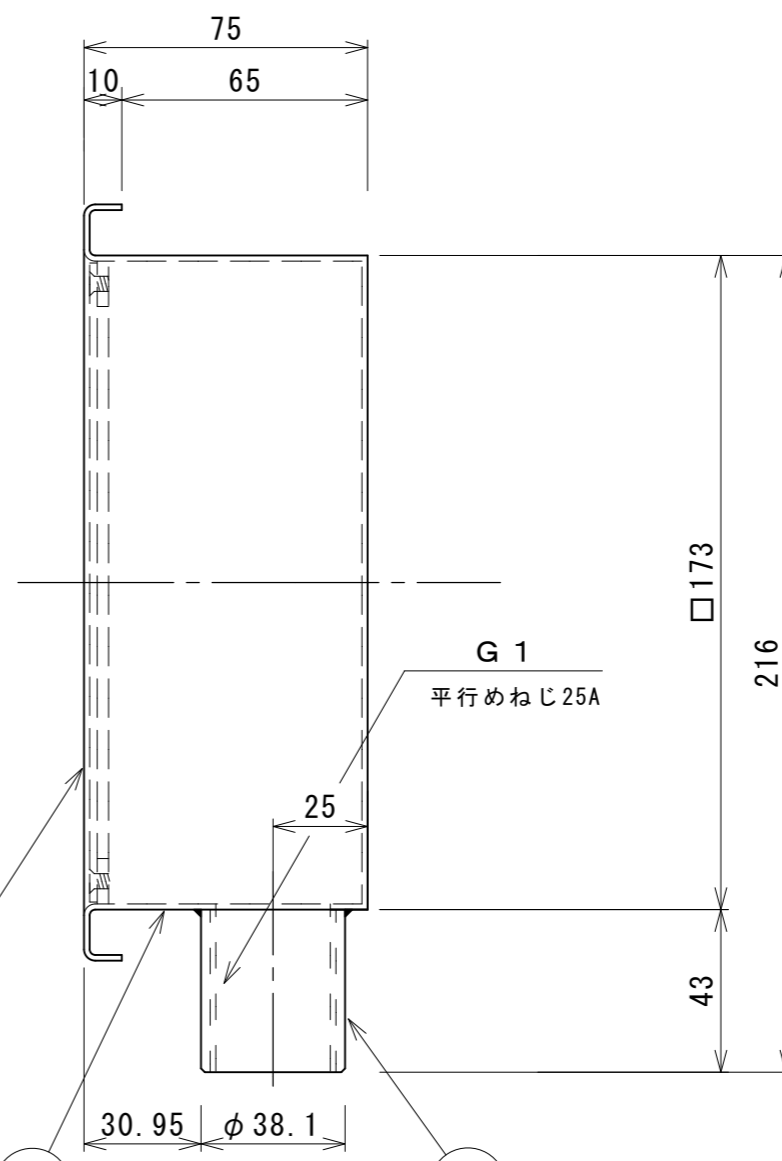
断側面図
