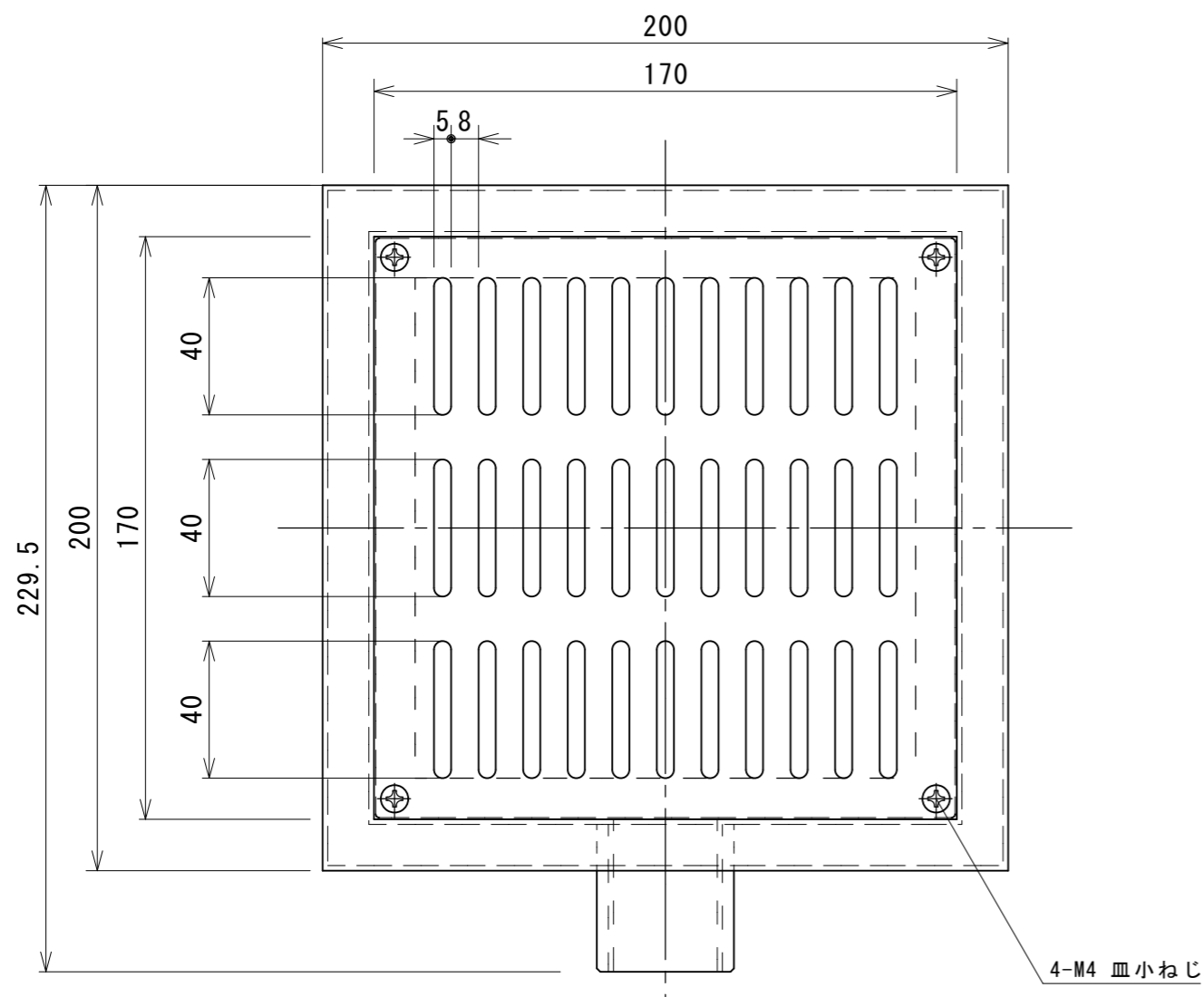
平面図
