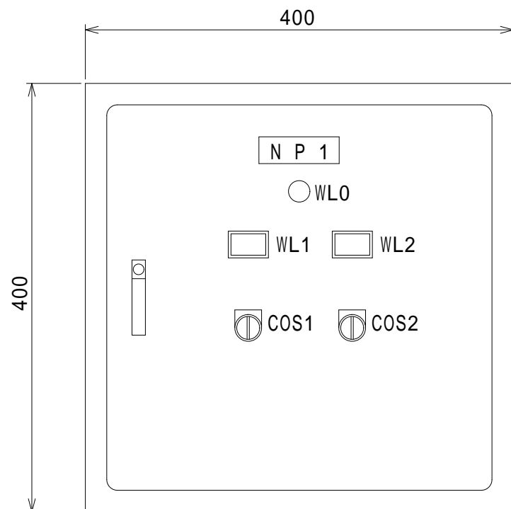
正面図
