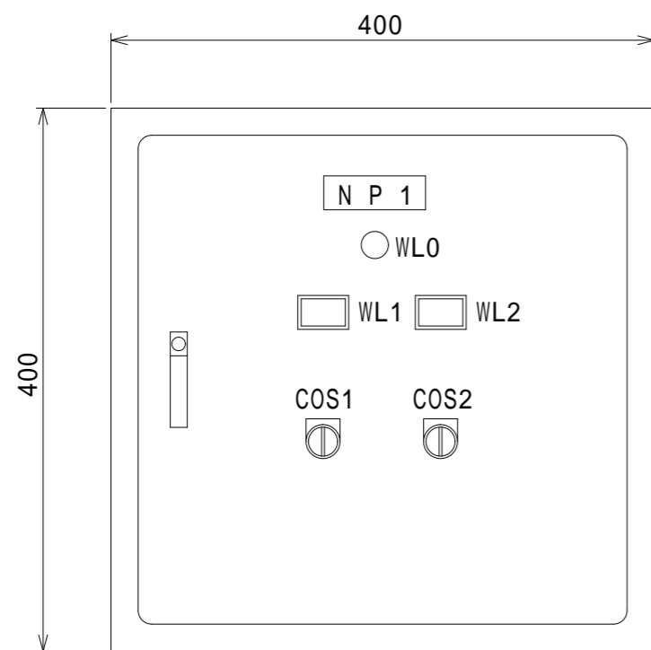
正面図
