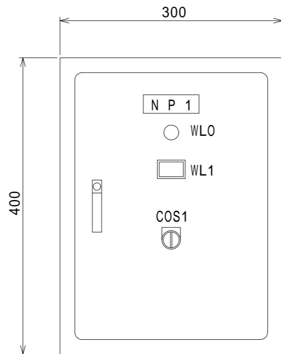
正面図
