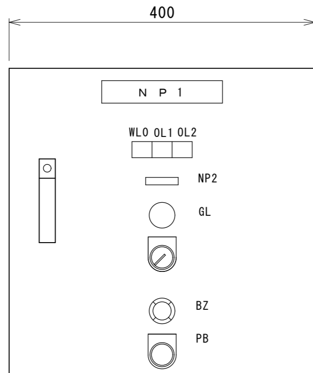
正面図
