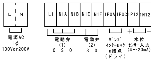
端子台図
