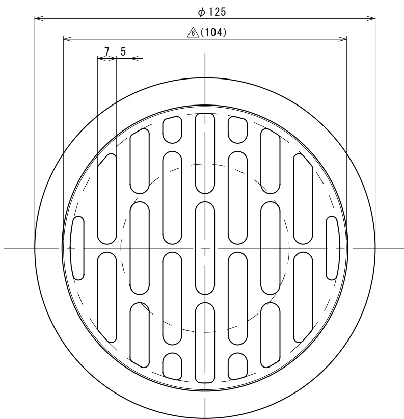
平面図
