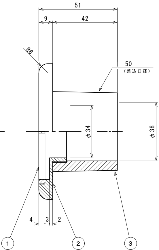
断側面図
