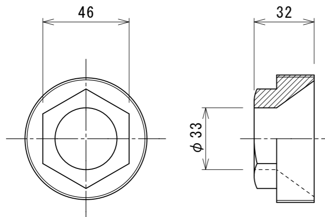
② オリフィス部品図
