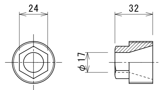
② オリフィス部品図
