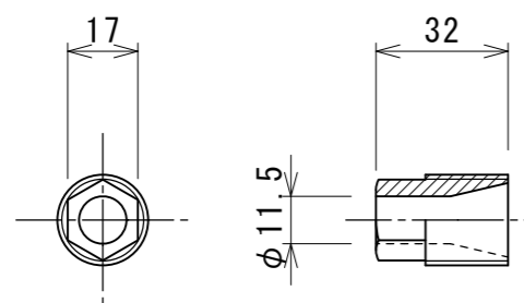
② オリフィス部品図
