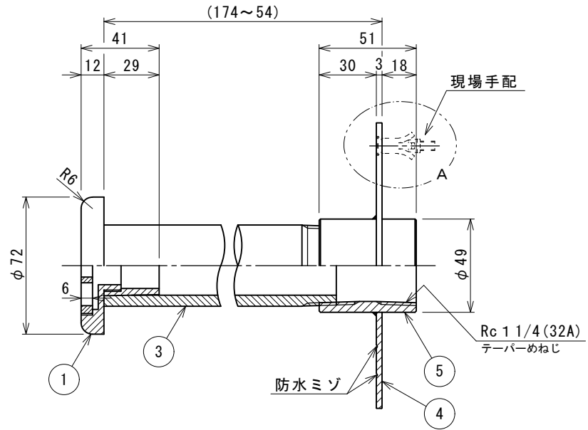
A部施工例 S=NON (a)及び(b)は現場手配
