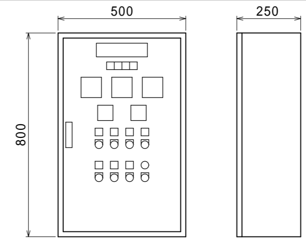
②④ 制御盤 屋内設置タイプ 60Hz用
