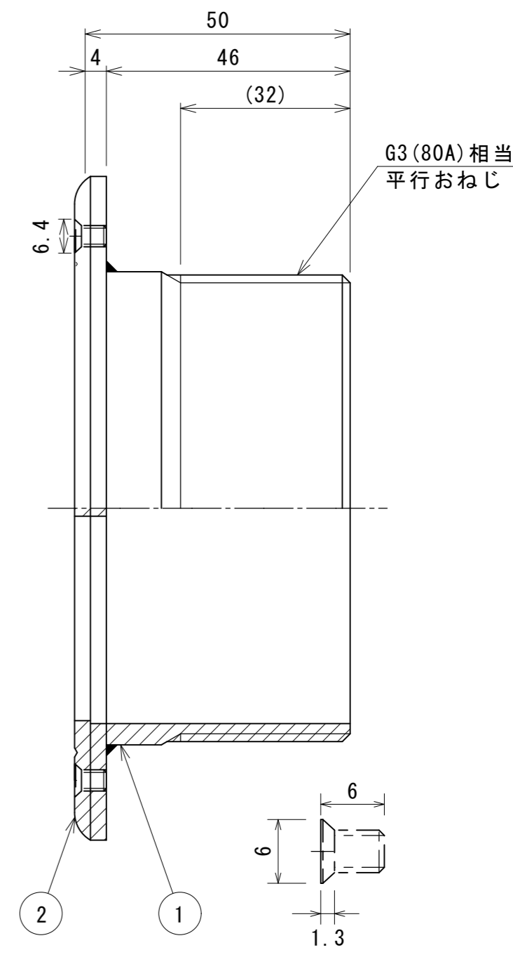
SNFS-SD M4×6L 固定ボルト詳細図 S=NON
