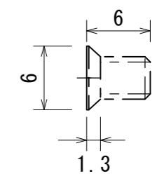
SNFS-SD M4 × 6L 固定ボルト詳細図 S=NON
