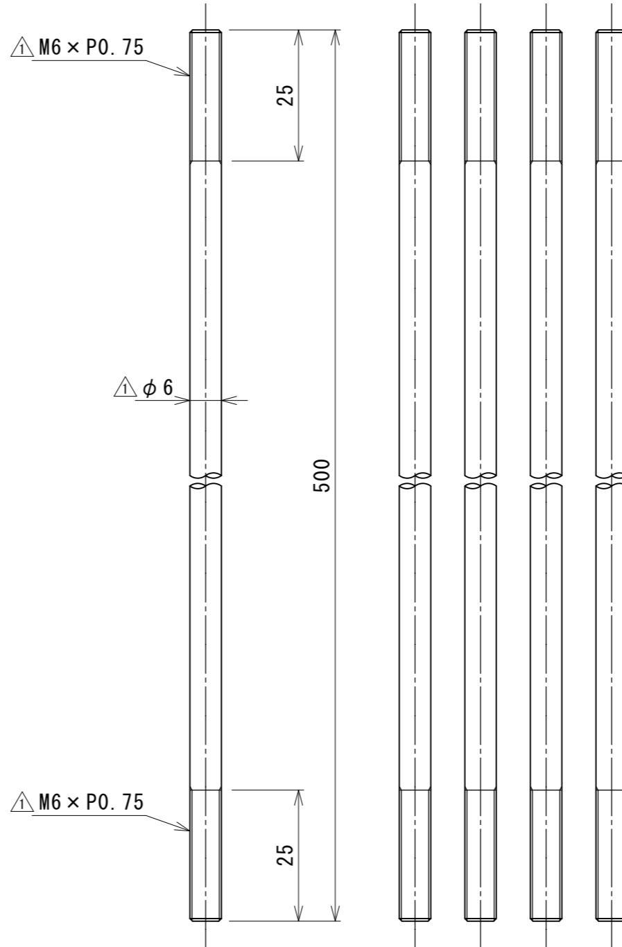
8 電極棒 S=1/1
