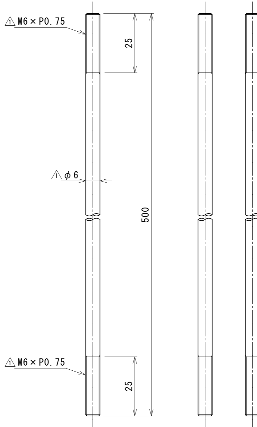
8 電極棒 S=1/1
