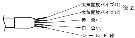
A部ケーブル接続図 S=NON
