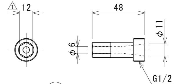
3 内部ノズル
