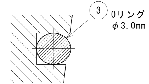
A部詳細図 S=5/1
