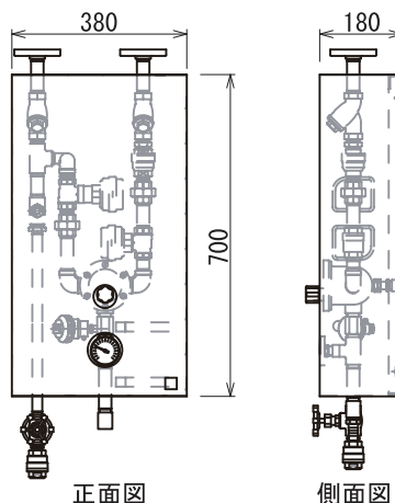
FSD-20S取付イメージ
