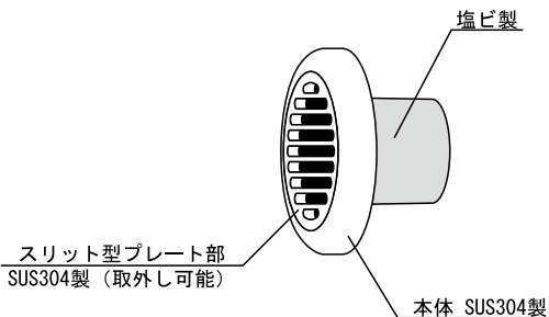
本体 SUS304製
