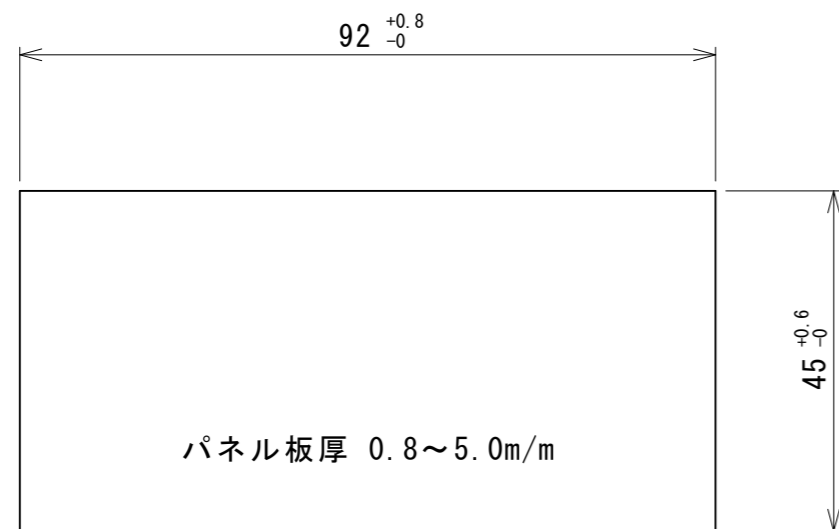
パネル切穴
