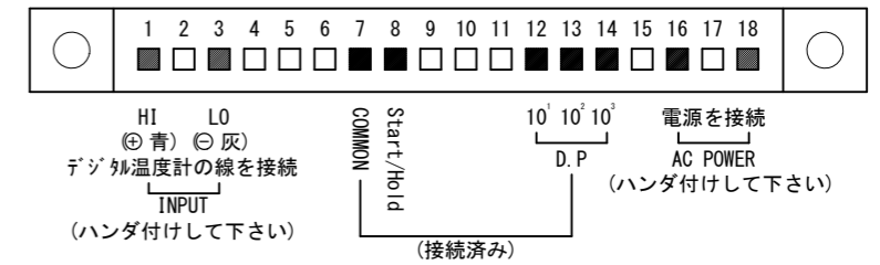
端子台図
