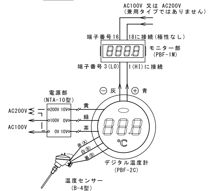
結線図
