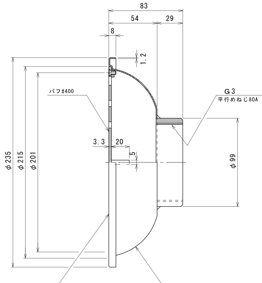
断側面図
