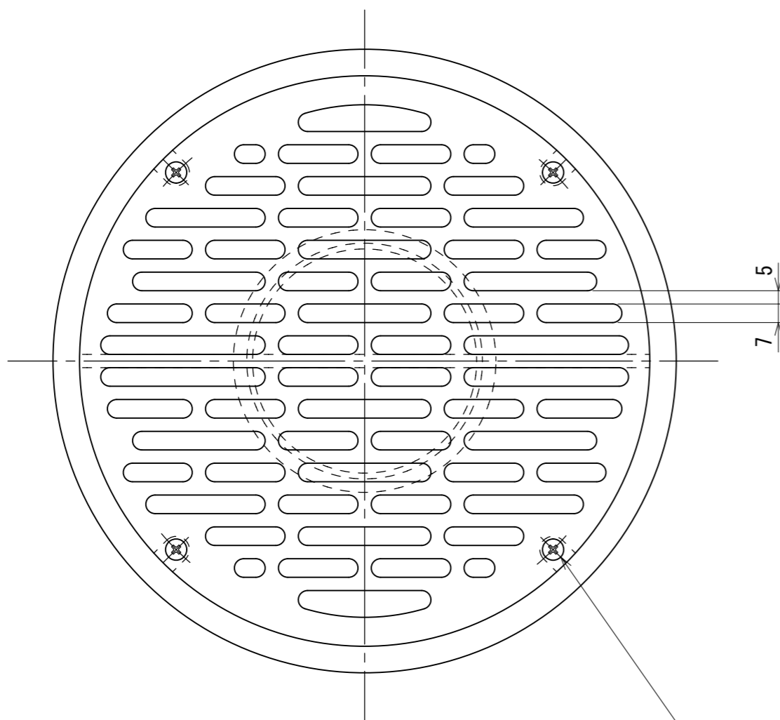
平面図
